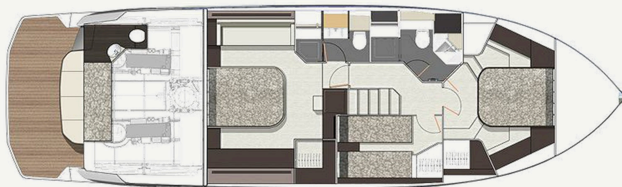
Нижняя палуба · 3 каюты + каюта экипажа
