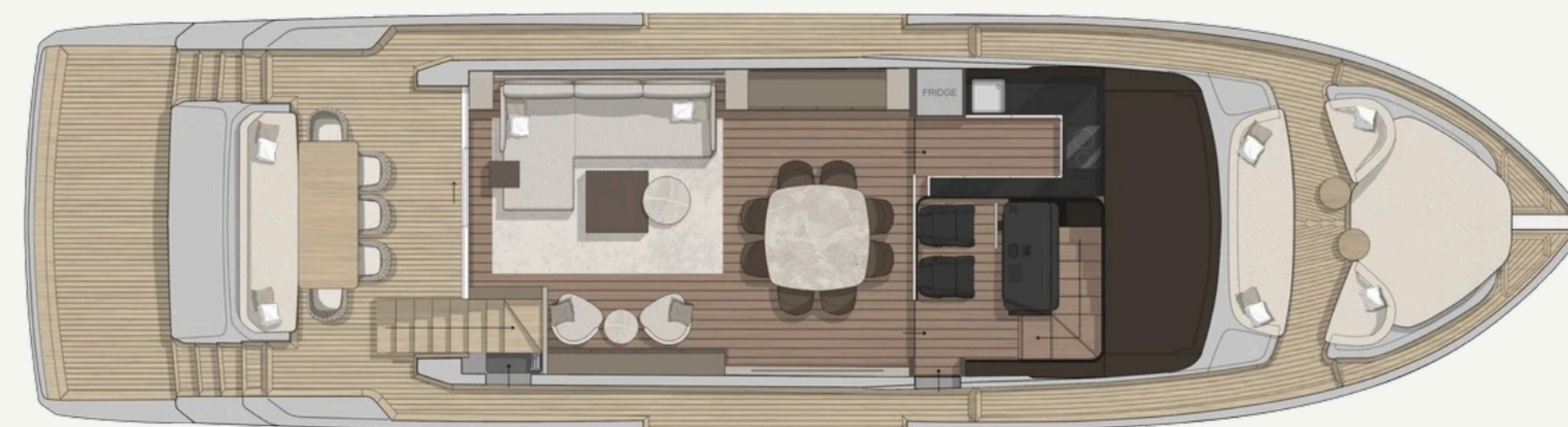
Главная палуба
